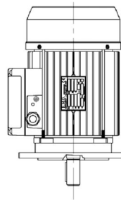
IM V18
